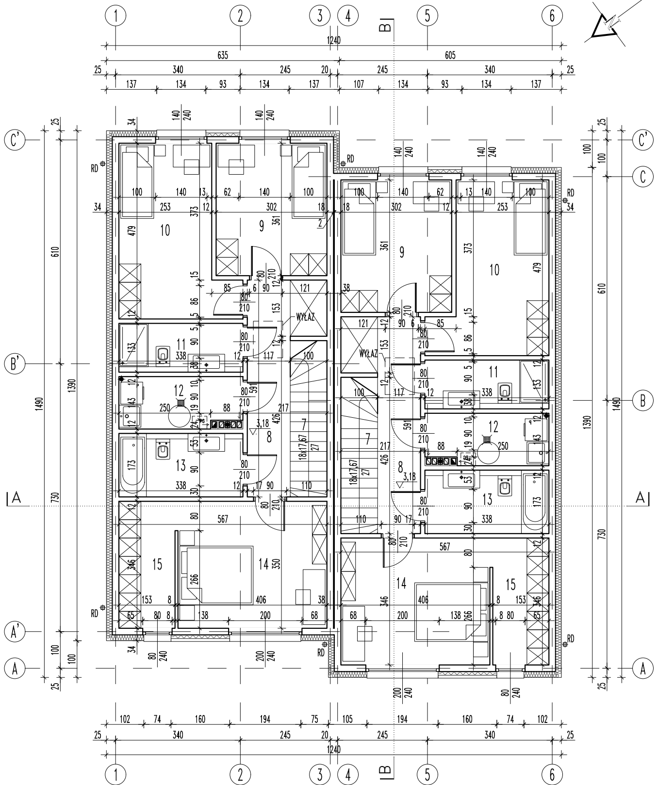
RZUT PIĘTRA, SKALA 1:100
